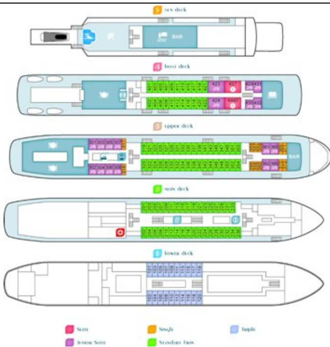
Planimetria motonave Bulgakov
